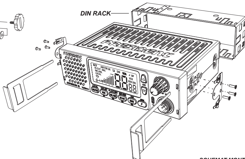
SCHEMAT MONTAŻU
