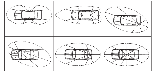
LOBE DE RAYONNEMENT
